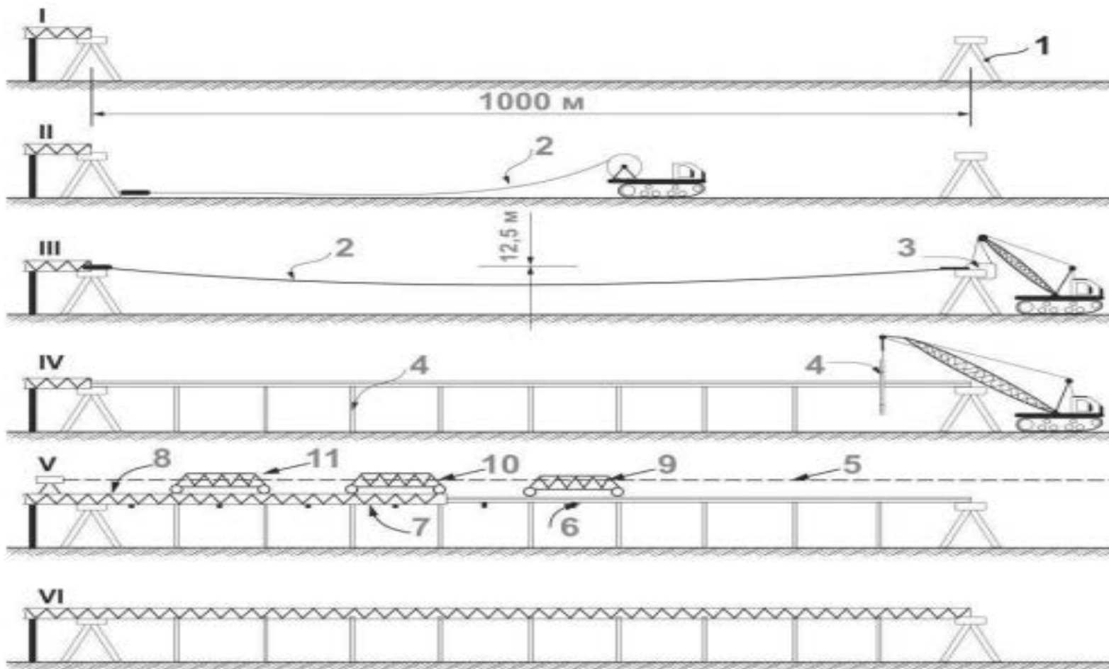
Рис. 41. Технология строительства трассы SkyWay (вариант):
